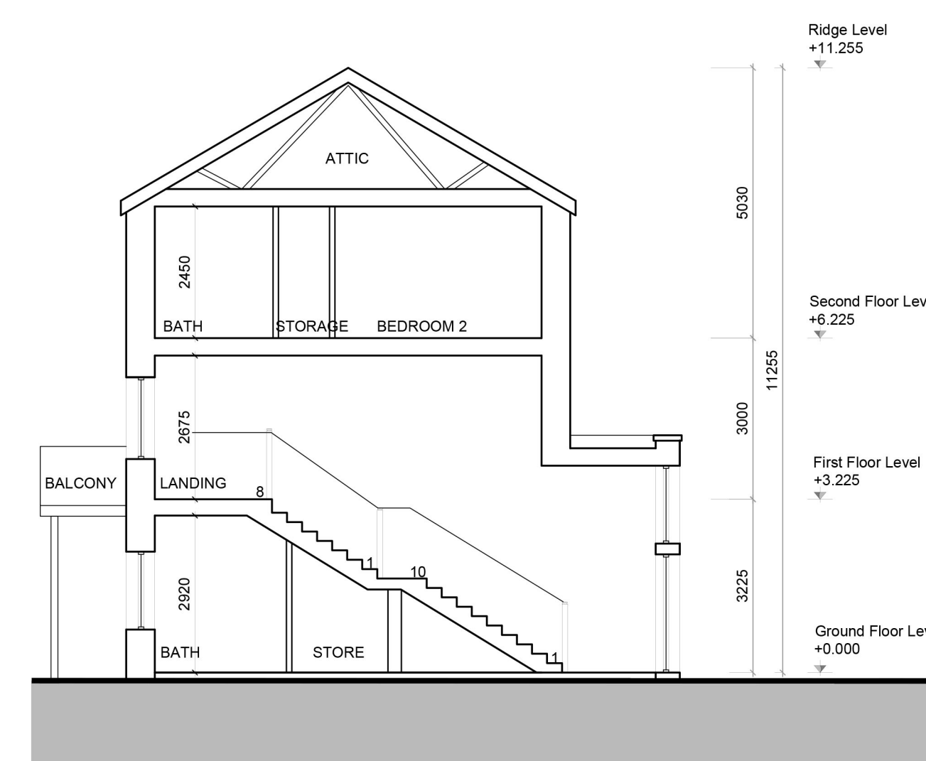
SECTION A-A
